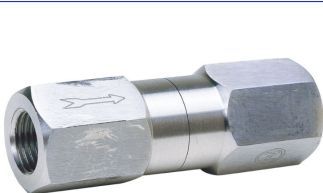
inox terugslagklep PN16 met flapper / zonder veer fig 712 : FF 1/2" - 2" bsp teflon klepring temp. : -30°C +180°C max. 16 bar bij 120°C max. 10 bar bij 180°C fig 712NPT : met NPT draad
